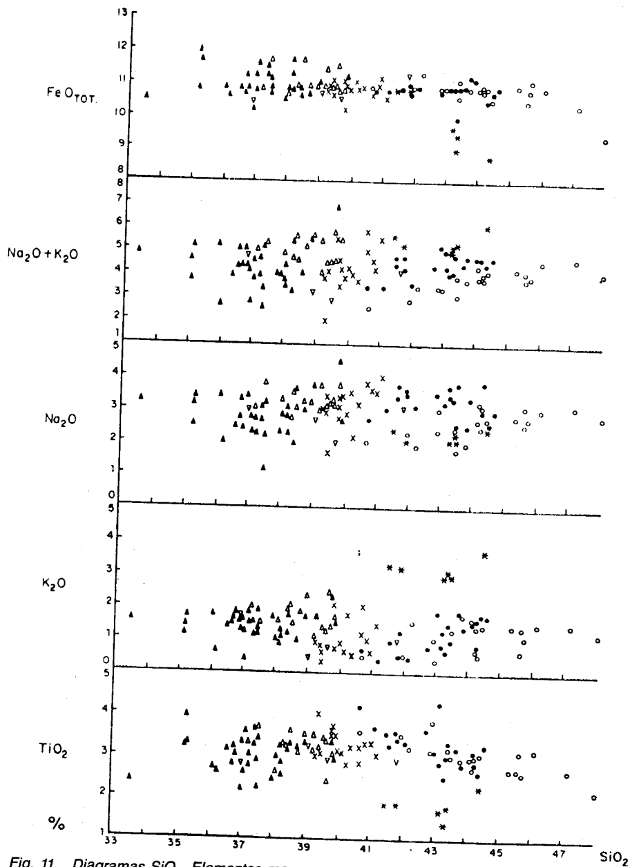
Fig. 11. Diagramas \text{SiO}_2 . Elementos mayores.
