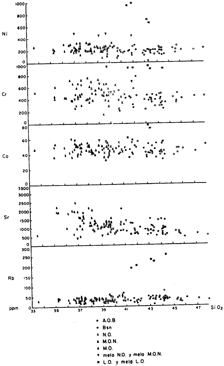
Fig. 8. Diagramas \text{SiO}_2 . Elementos menores.
