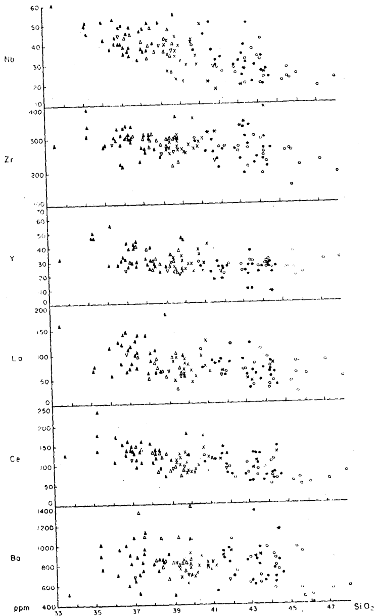
Fig. 9. Diagramas SiO 2 . Elementos menores.
