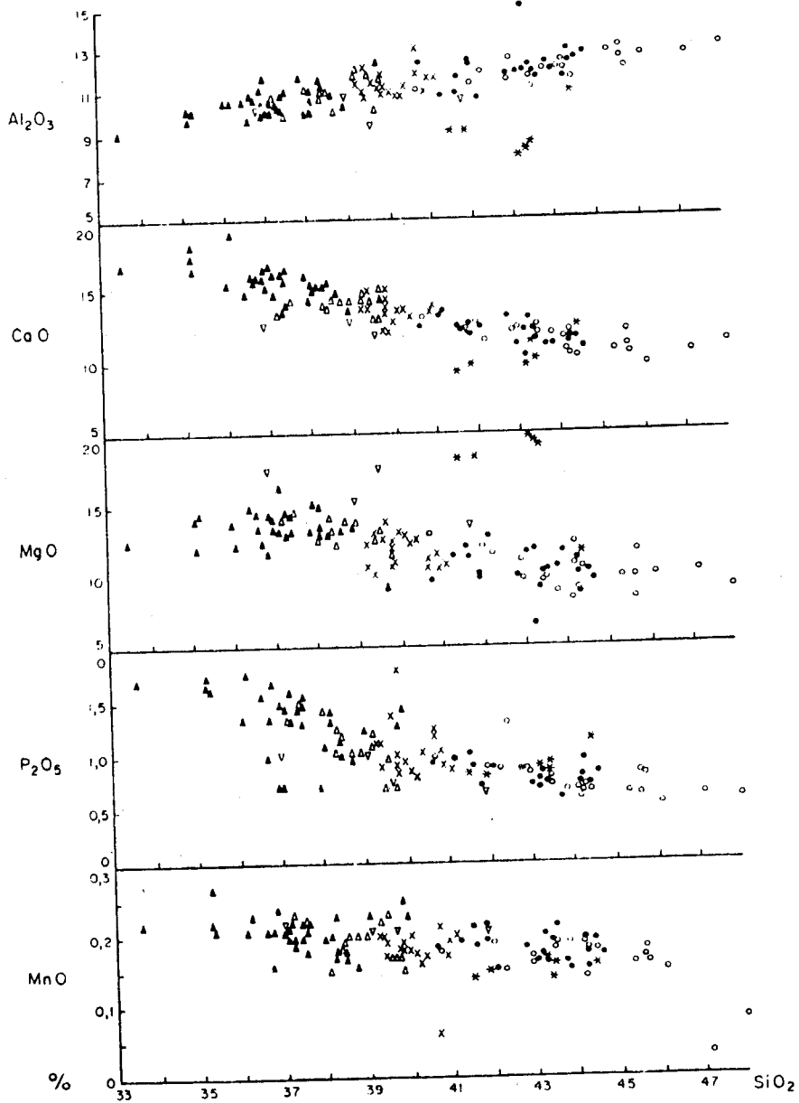
Fig. 10. Diagramas \text{SiO}_2 . Elementos mayores.
